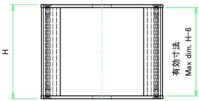
Wパネル1 / W Panel 1
